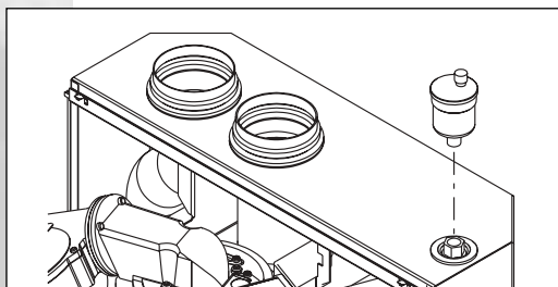
Figuur 14: Montage automatische ontluucher
