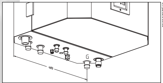
Figuur 16: Gasleidingaansluiting
